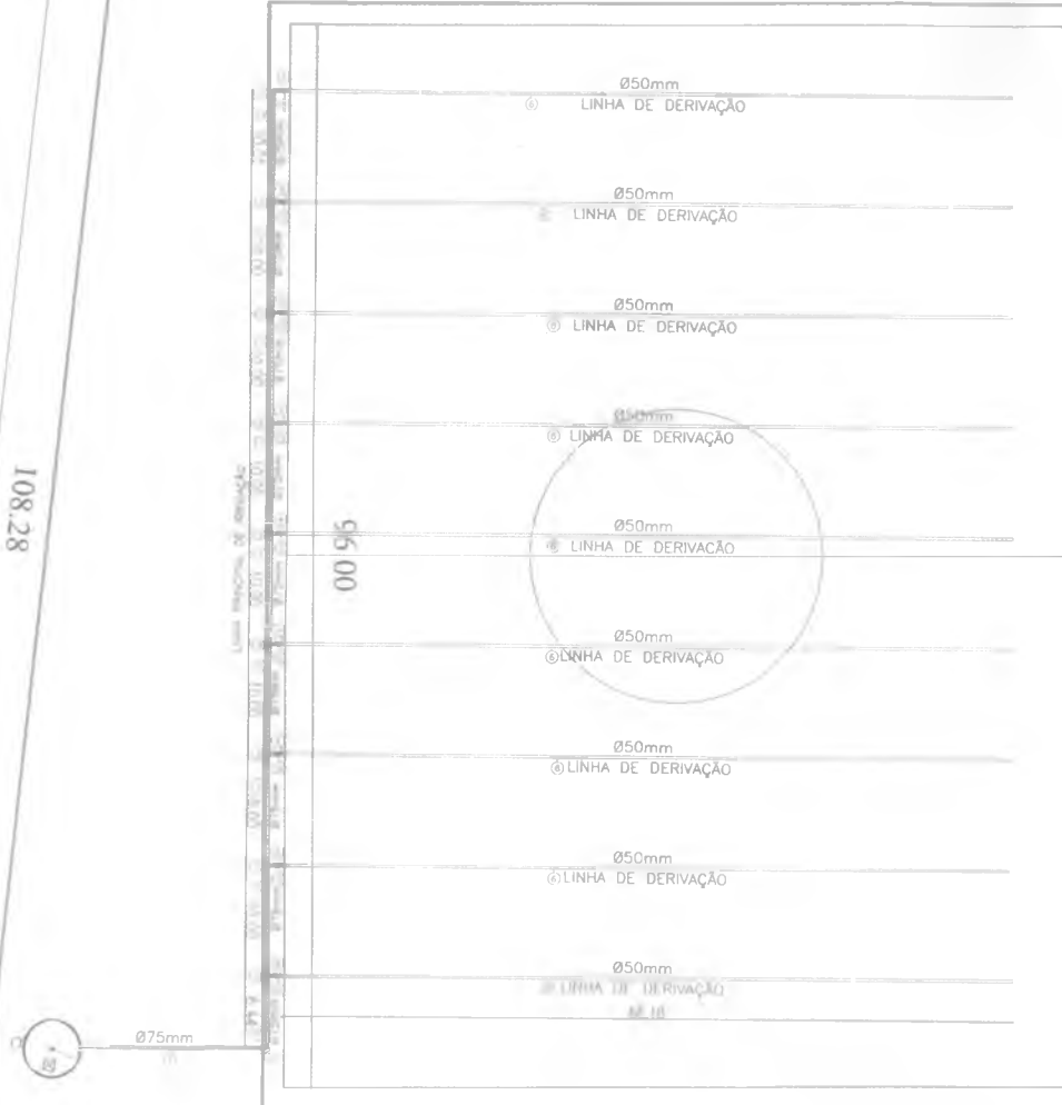
01 PLANTA DRENAGEM
